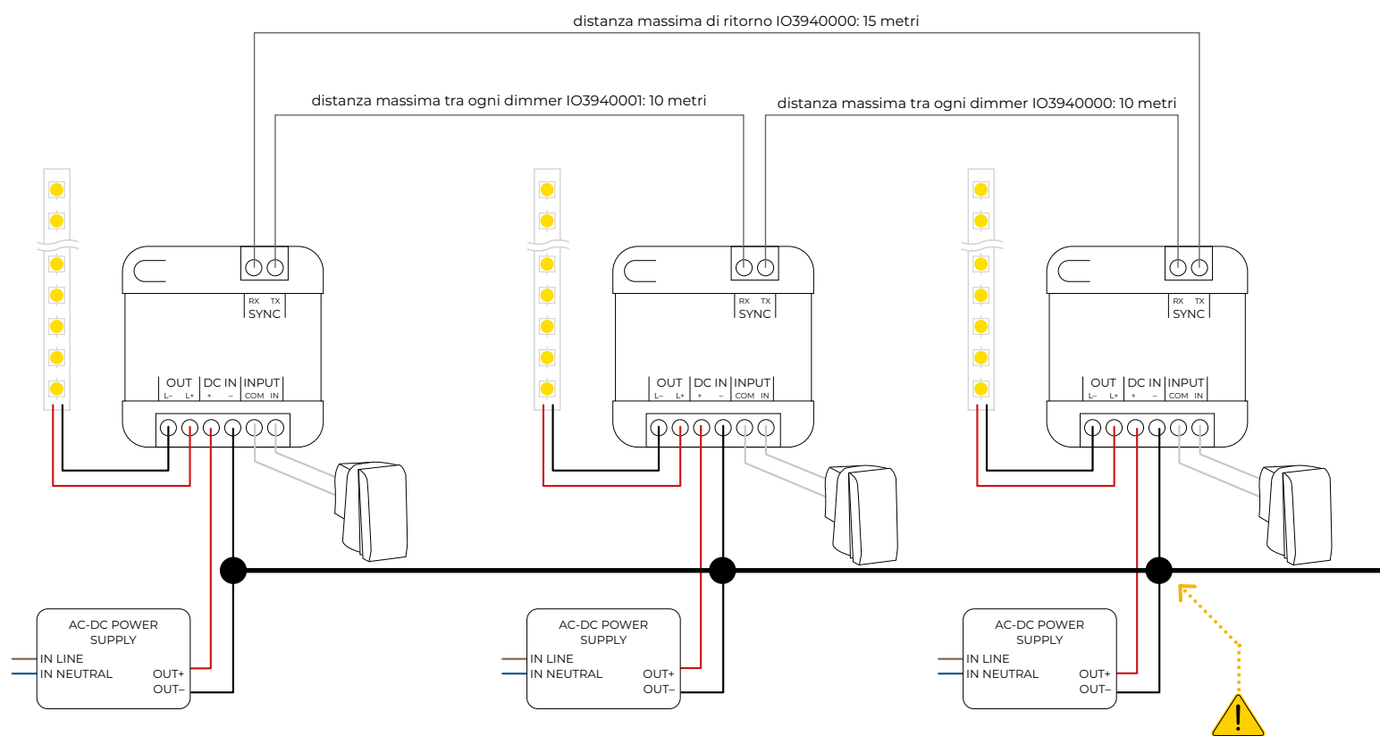
FIG. 9 - collegamento sincronizzazione multi-master alimentatore multiplo PUSH-CV
