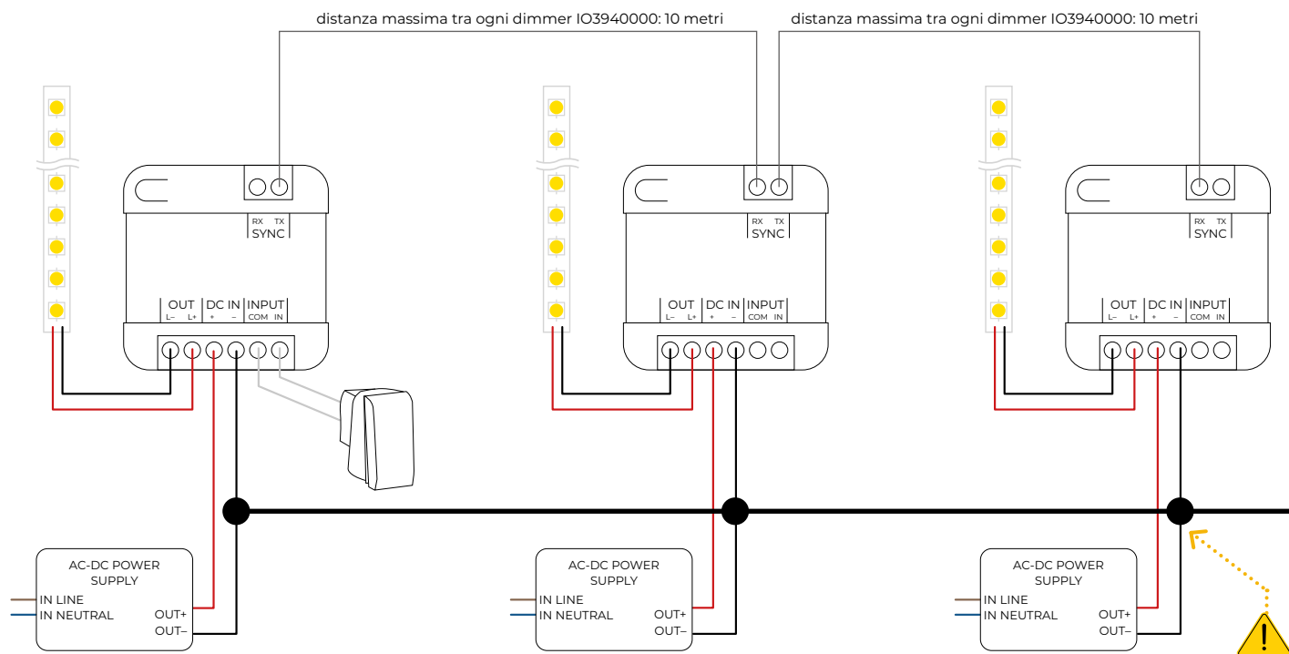
FIG. 7 - collegamento sincronizzazione schema 2 IO3940000 alimentatore multiplo
