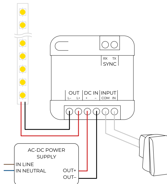
FIG. 1 - collegamento pulsante IO3940000
